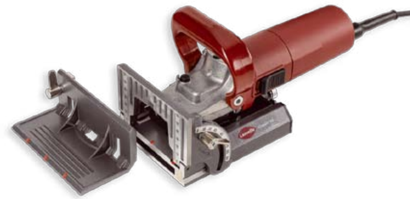
Ensamblaje con laminas de madera
