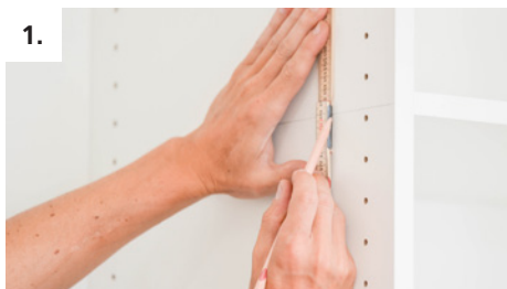
1. Mittenposition des Fachbodens auf den Korpusseiten anreissen
